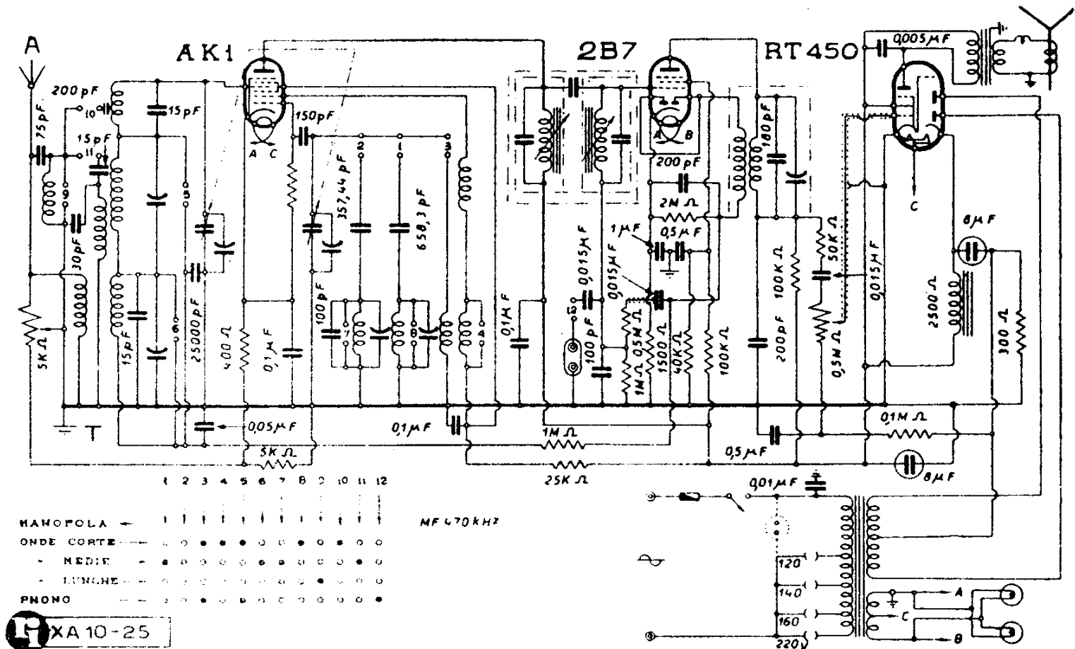
E.M.I. - MOD. PHONOLA « 650 B »
